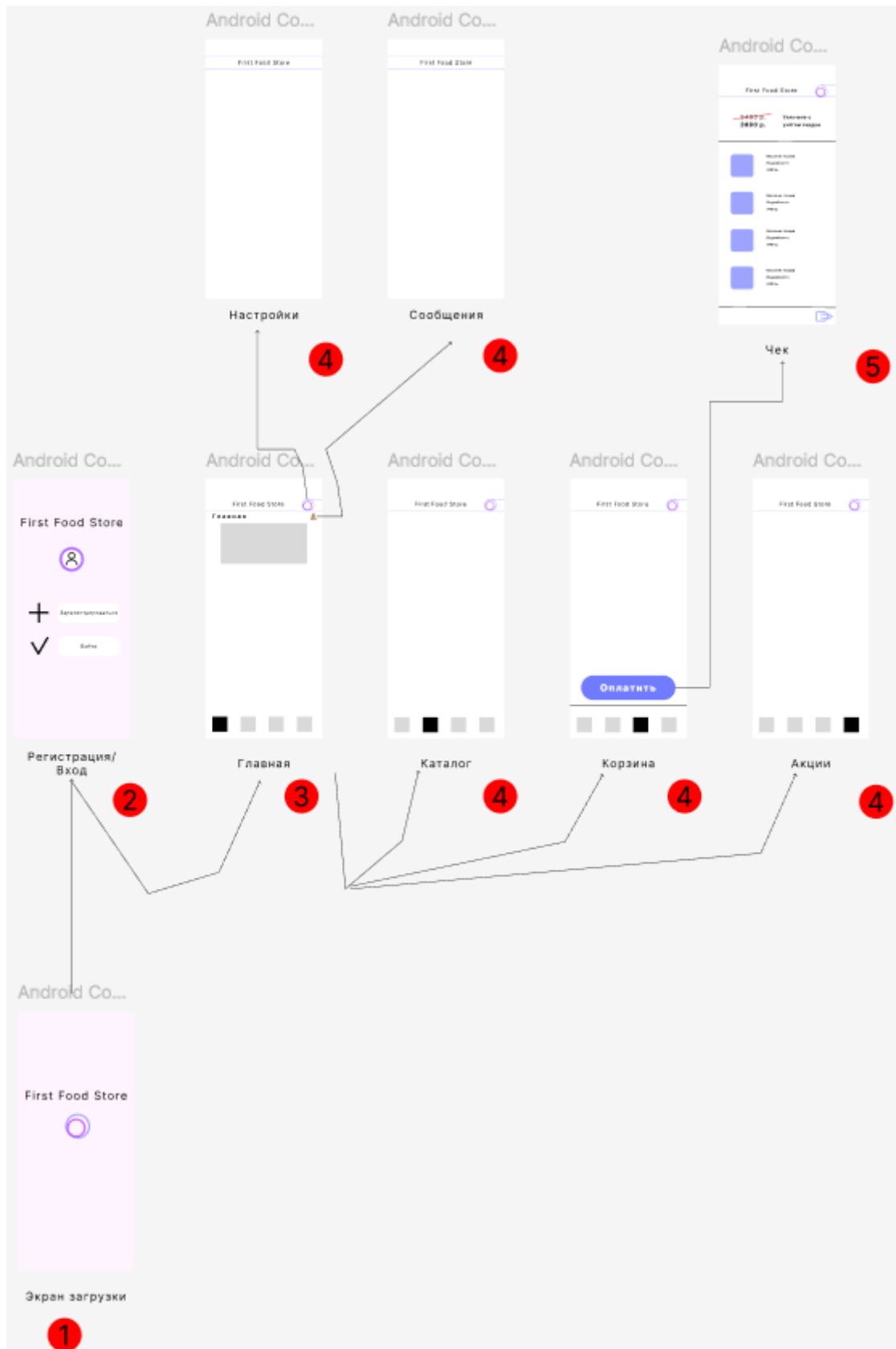
Рисунок 2 – Карта интерфейсов системы.
